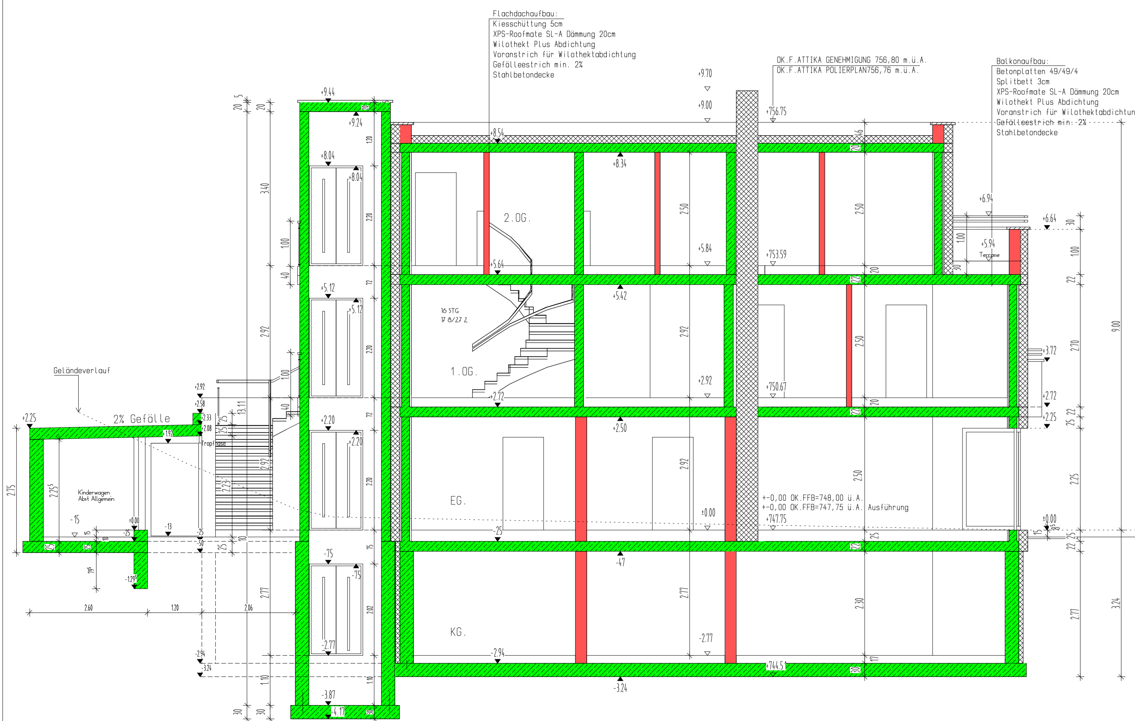
SCHNITT A-A
