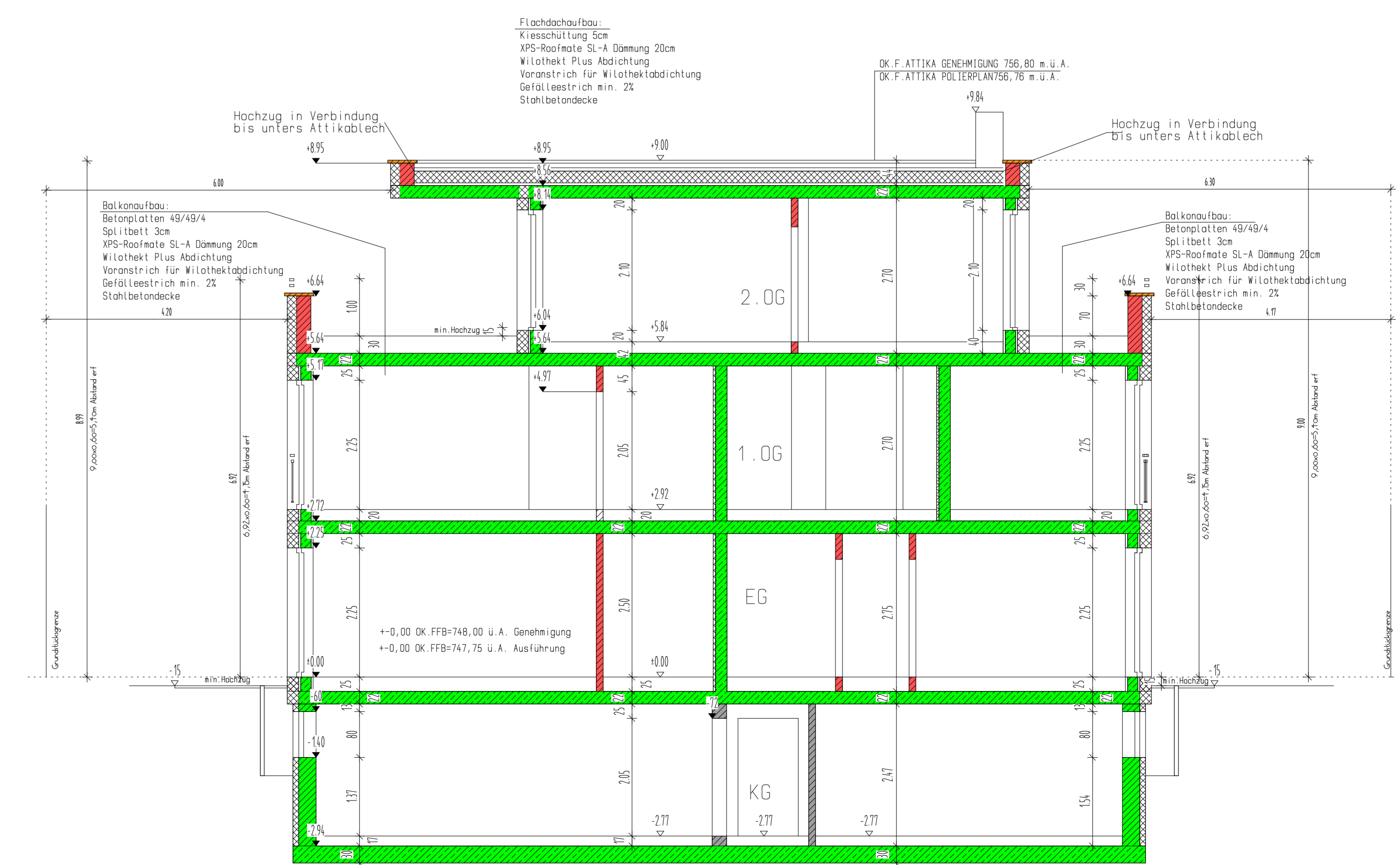
SCHNITT E-E
