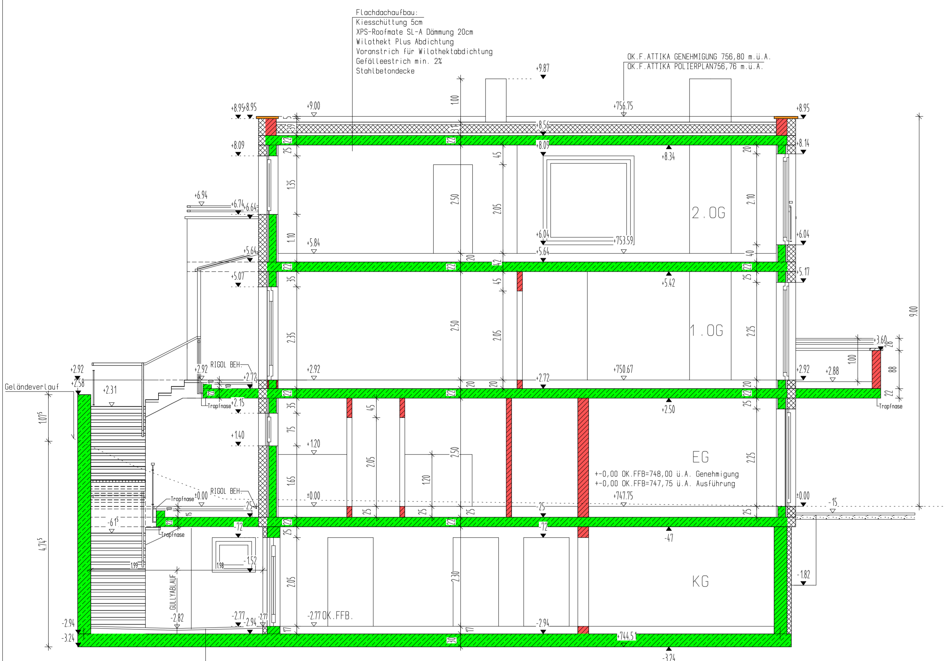
SCHNITT B-B
