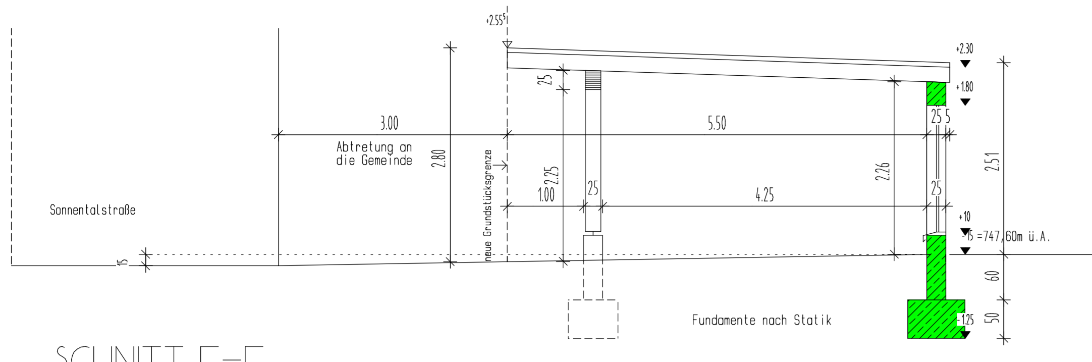
SCHNITT F-F
