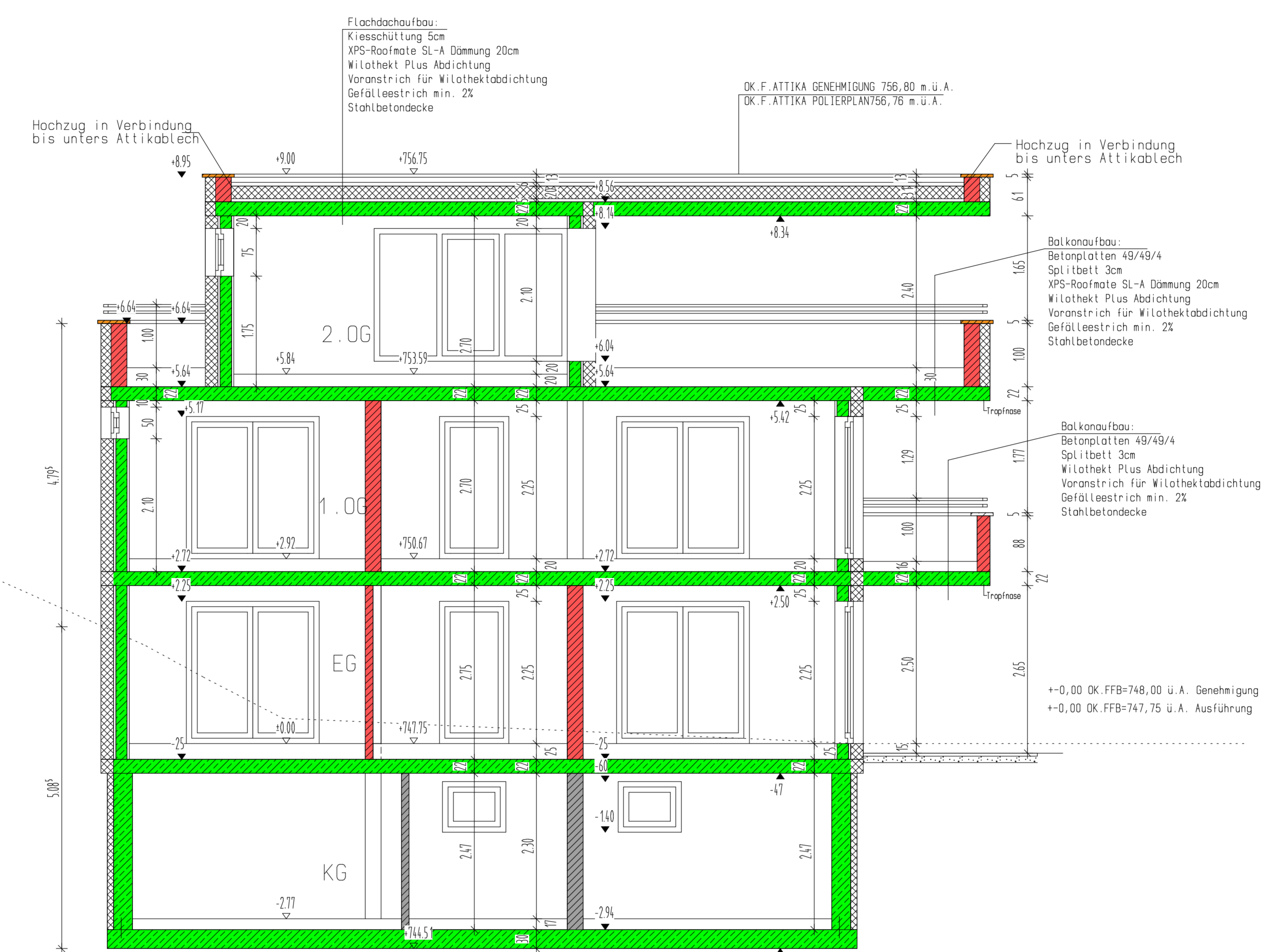
SCHNITT C-C
