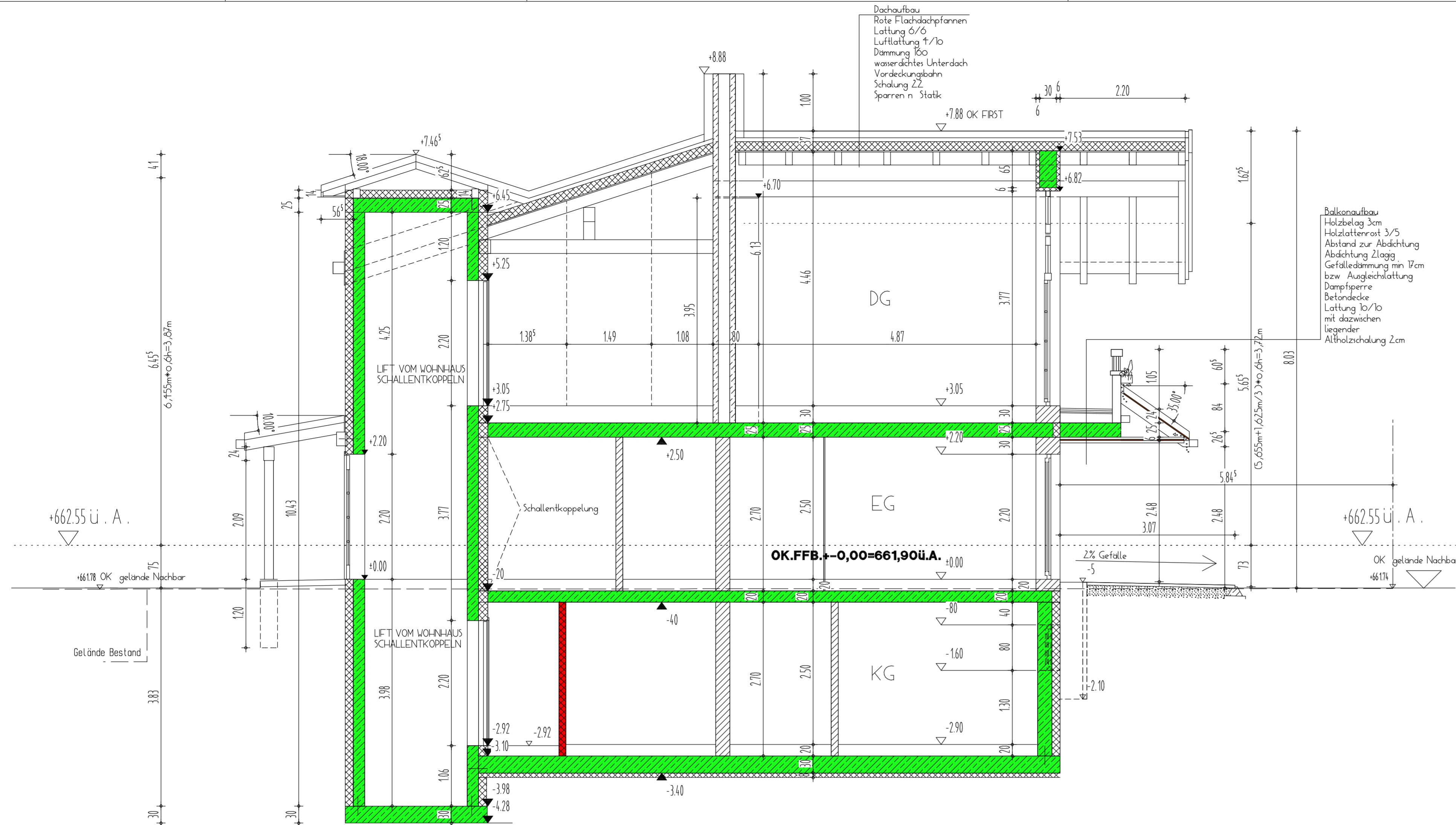
SCHNITT A-A
