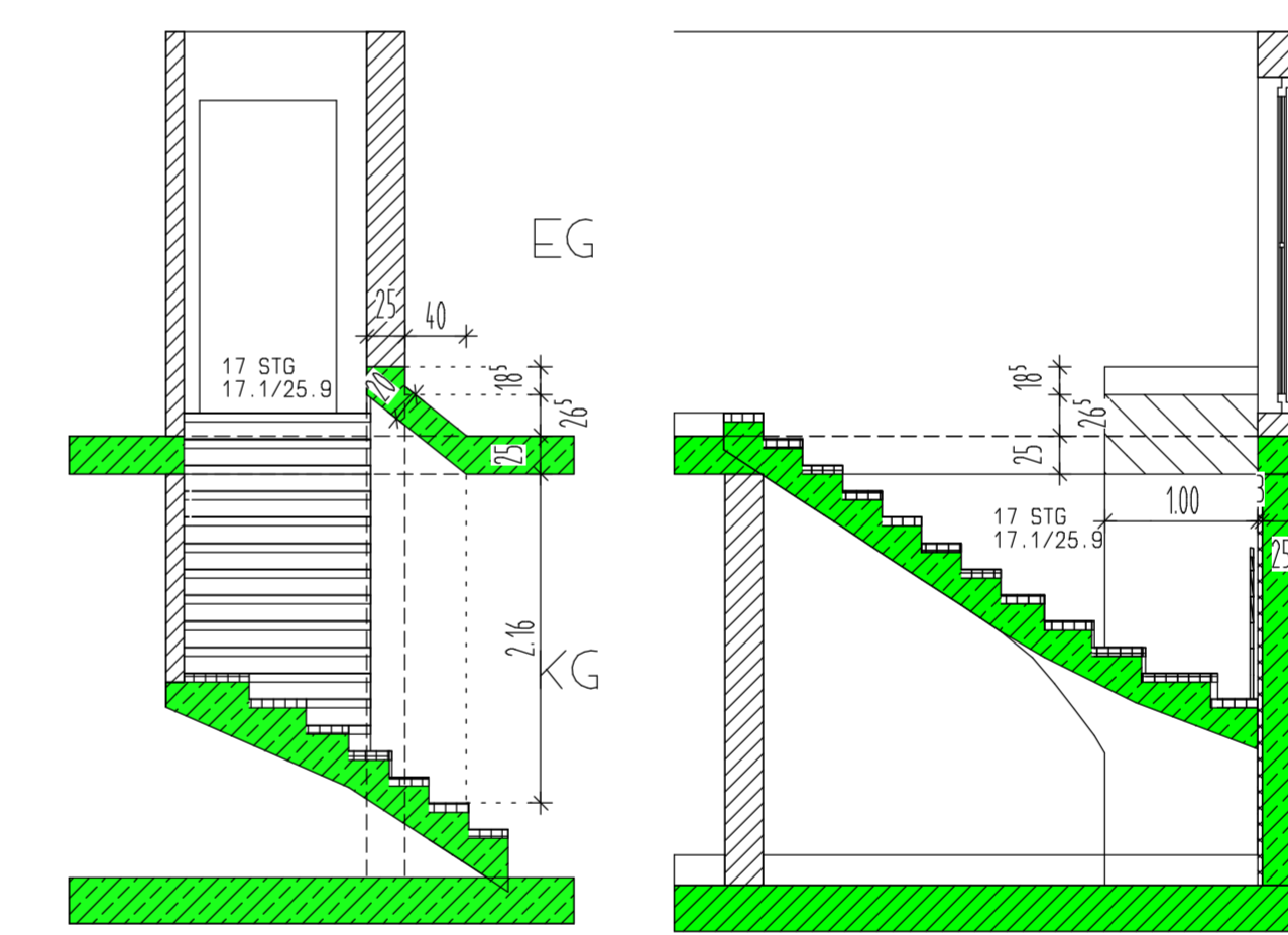
SCHNITT T-T WOHNINGSTREPPE
