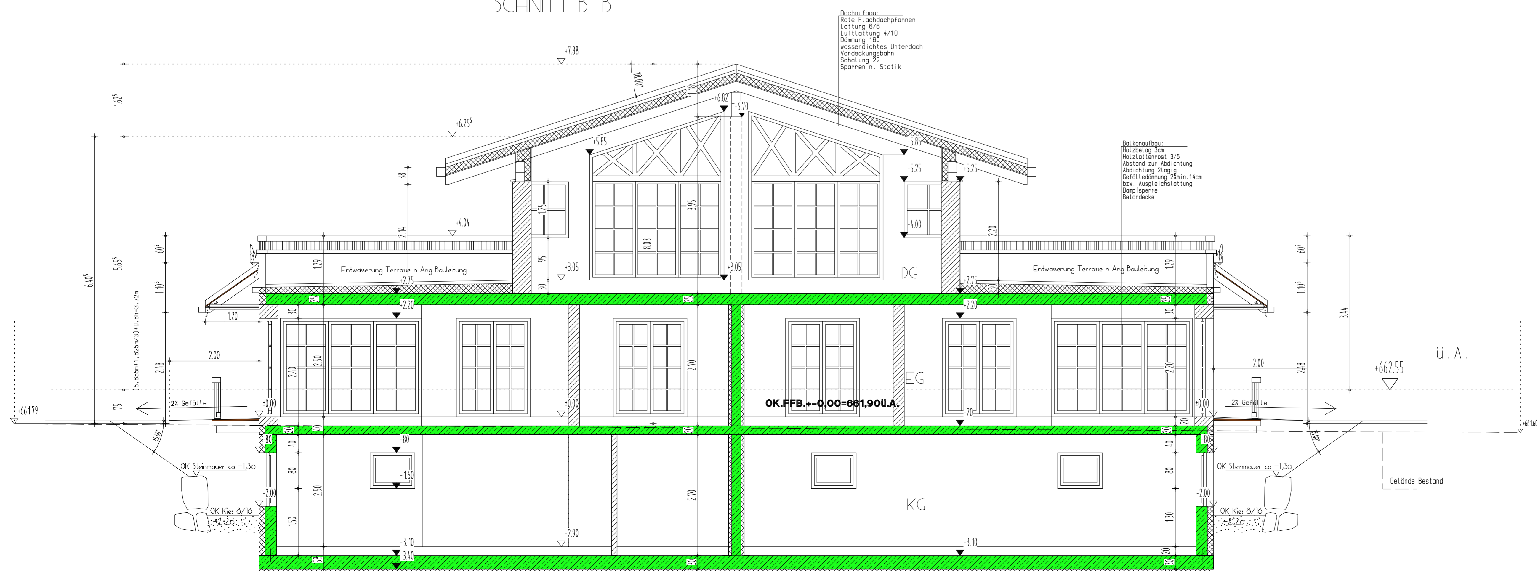
SCHNITT C-C
