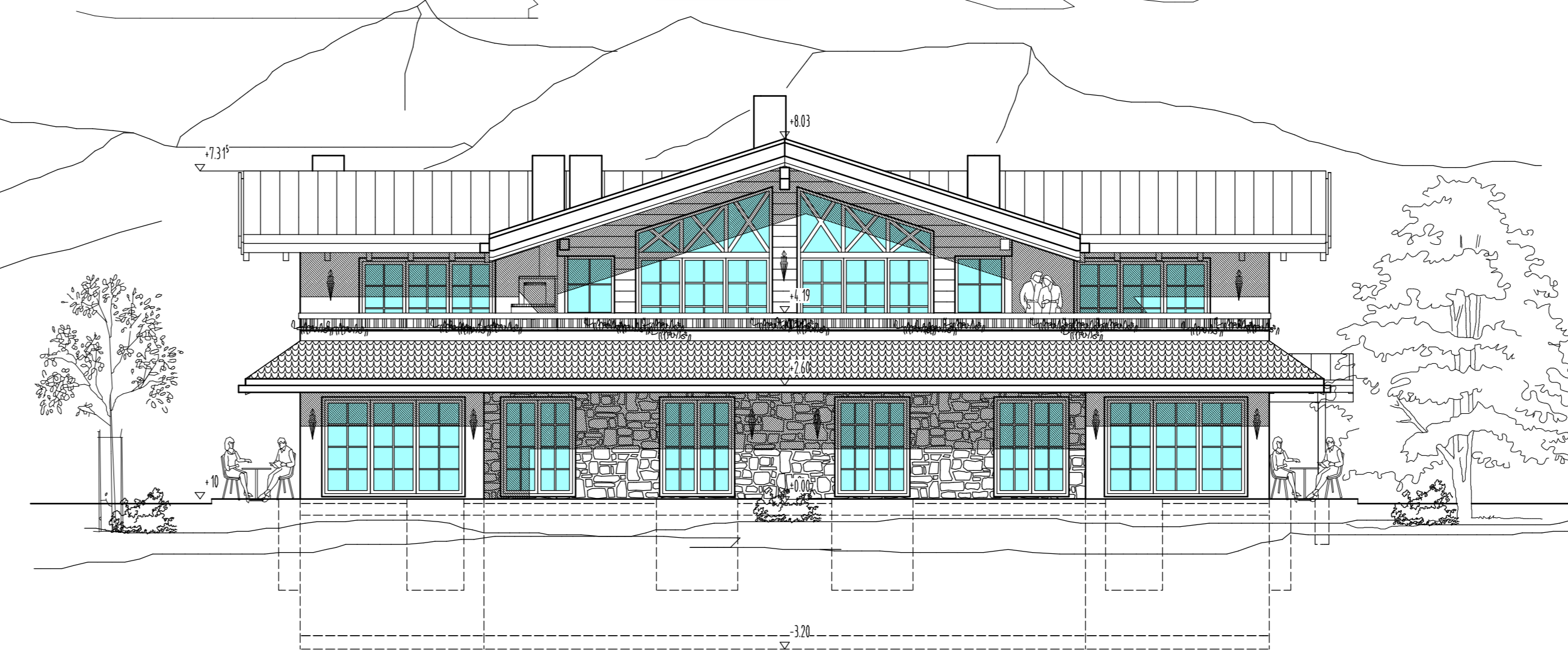
SUDWESTANSICHT
