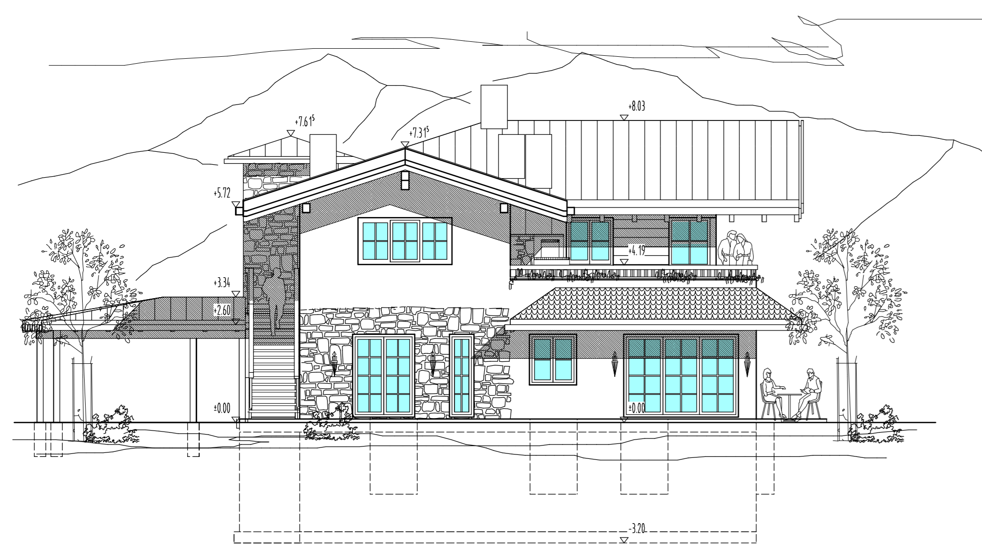
NORDWESTANSICHT
