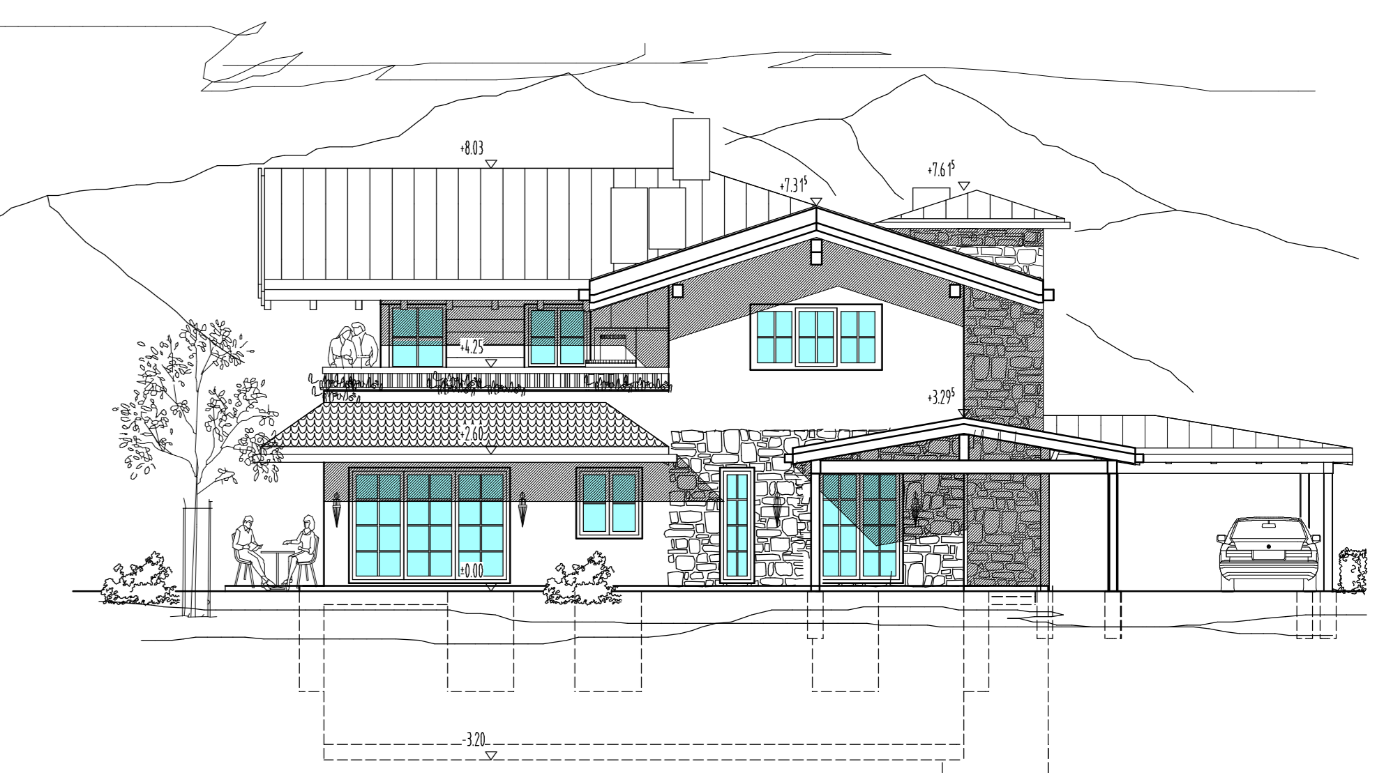
SUDOSTANSICHT
