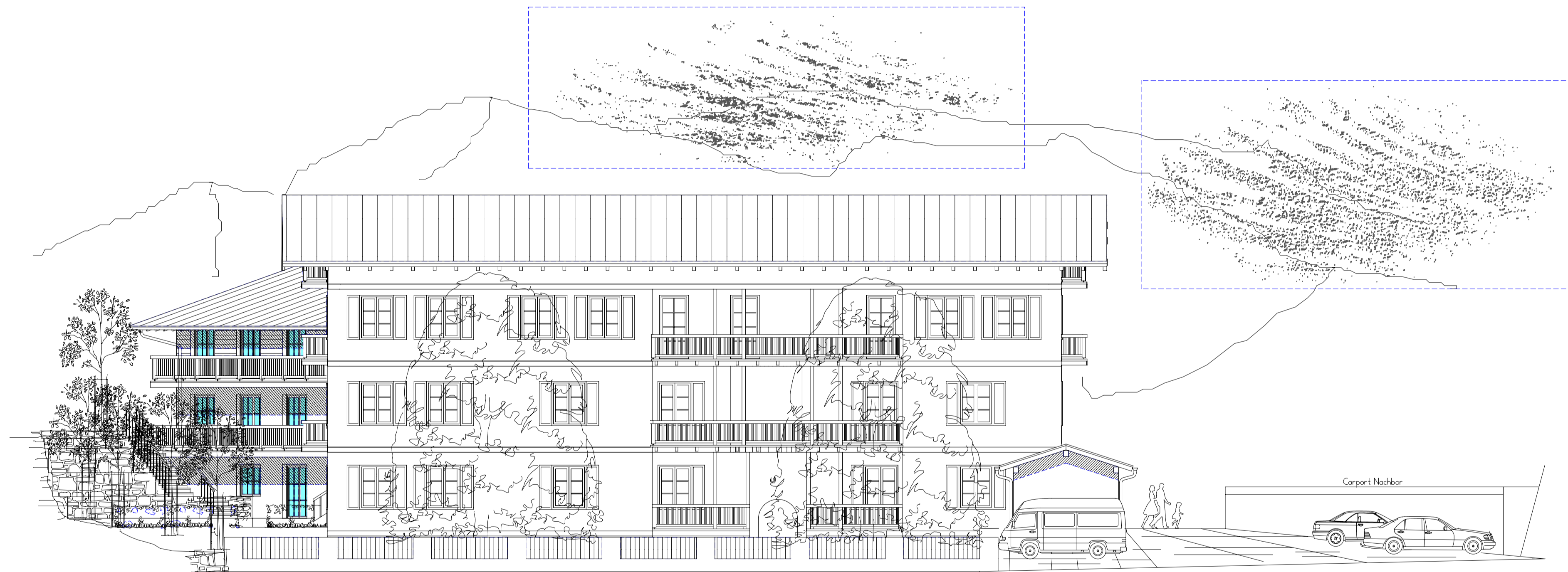
SÜDANSICHT von der Tiroler Straße
