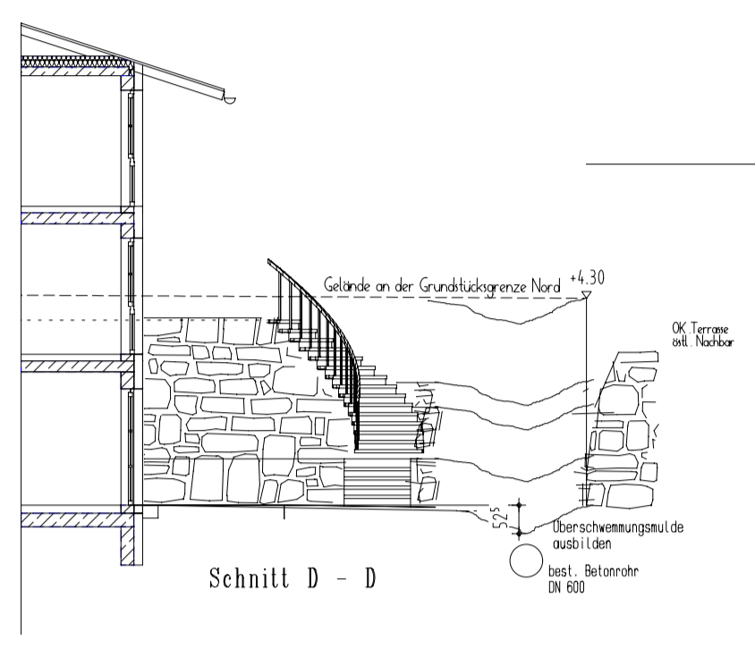
Wasserüberlauf am Bauhofer Graben:
